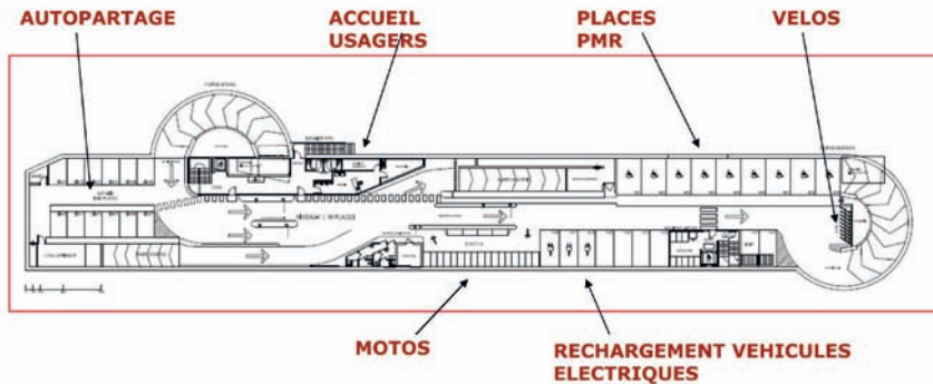
Plan-projet du niveau du Parking Bac-Montalembert
