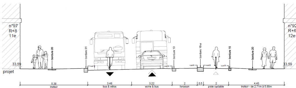
COUPE DE PRINCIPE DU PROJET FUTUR
