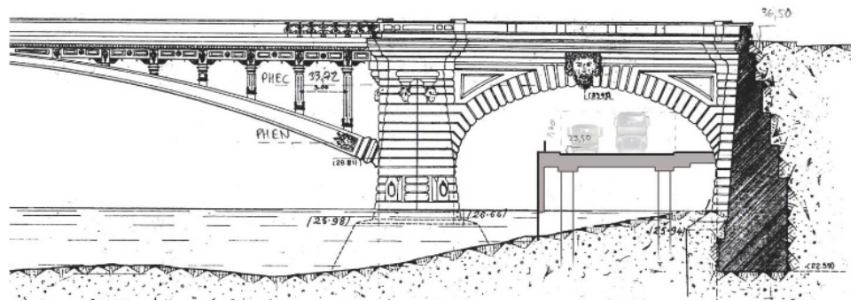
Figure 35 : Coupe de la structure des quais en amont du pont Notre-Dame Source : Mairie de Paris, Aménagement des berges de Seine rive droite, Voie Georges Pompidou
