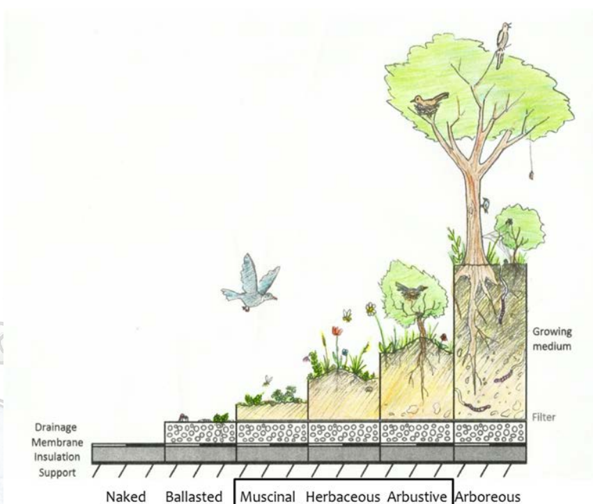
Figure 43 : Typologie des toitures végétalisées basées sur la structure de la végétation
