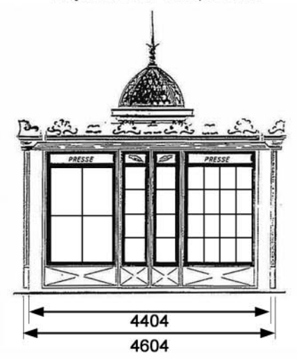
Façade Avant / Kiosque fermé
