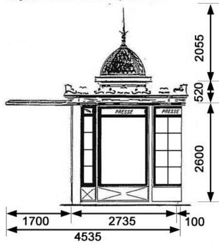
Façade Latérale / Kiosque fermé
